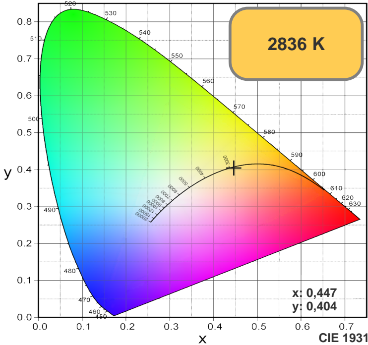
TM30: 77,8
