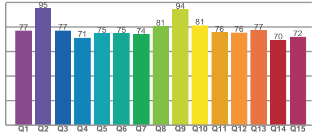
CQS: 76,9
