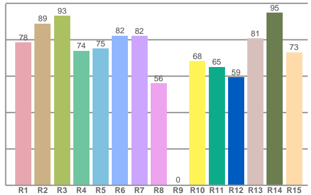
CQS: 76,9
