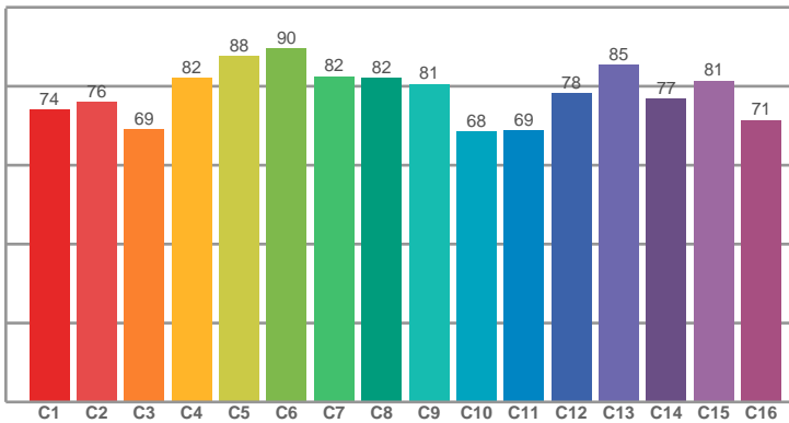
TM30: 77,8
